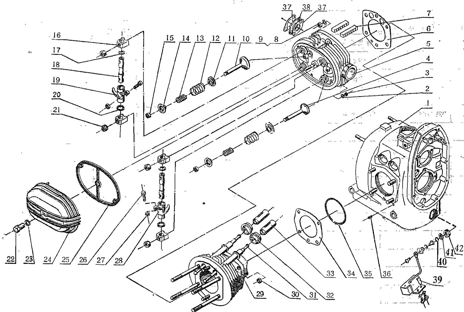
图17 F2P78FMF1b、L2P78FM 发动机（右侧视）
